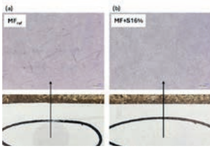
○ Vergleich der Laminatoberflächen nach Säurebehandlung: (a) beschädigte konventionelle MF-Oberfläche, (b) intakte Sorbitol-modifizierte MF-Oberfläche. Comparison of laminate surfaces after acid treatment: (a) damaged conventional MF surface, (b) intact sorbitol-modified MF surface.
