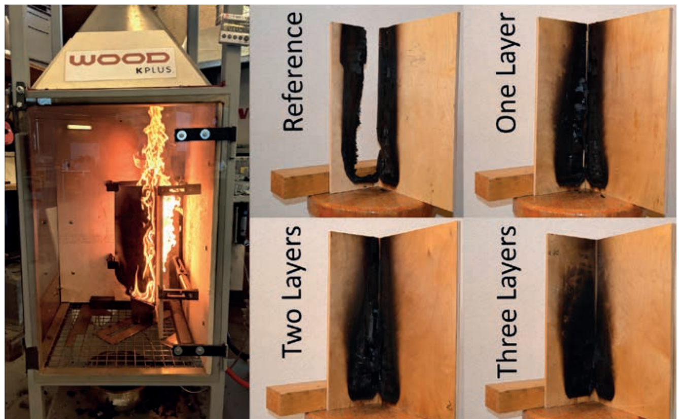
Brandversuch im Mini-SBI Test und Verbesserung durch heterogenen Aufbau Fire test in the mini-SBI test and improvement through heterogeneous design
