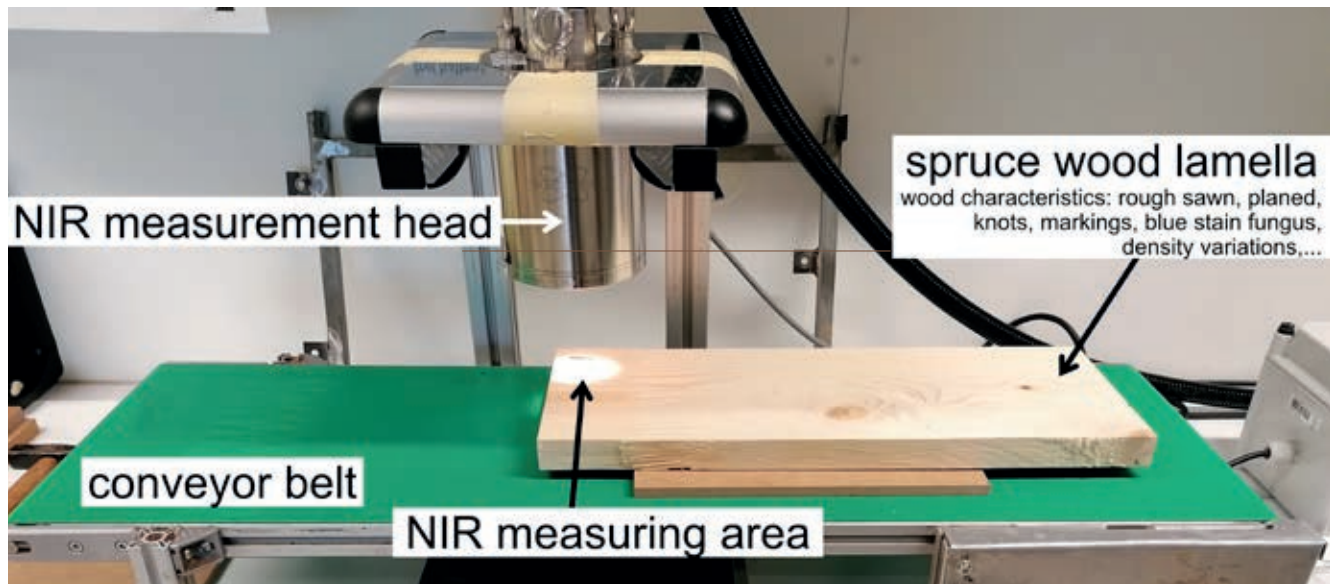
○ Prüfaufbau im Labormaßstab zur Messung der oberflächennahen Holzfeuchte an Fichtenholzlamellen mittels Nahinfrarotspektroskopie (NIR). Experimental setup on a laboratory scale for measuring the near-surface wood moisture of spruce wood lamella using near-infrared spectroscopy (NIR).
