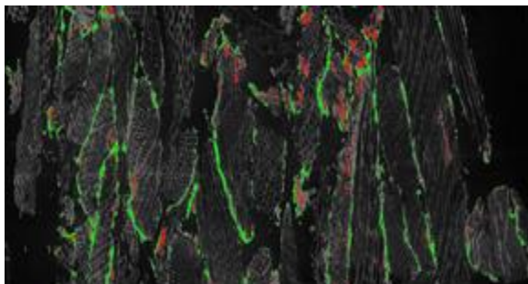
Abb. 2: Klebefuge (grün) und weggeschlagenes Bindemittel (rot) in der Spanplatte (Wood K plus)
